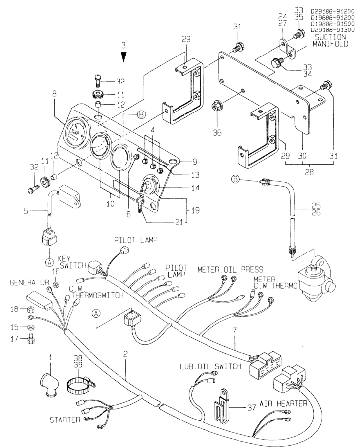
21. PANEL
