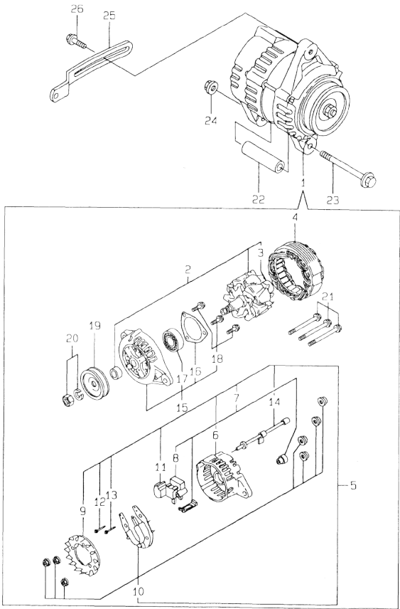
45. GENERATOR
